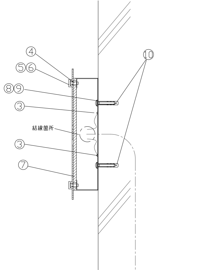
A-A拡大断面図(S=2/1)
